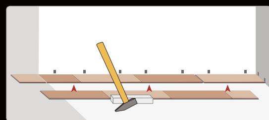
05 СОБЕРИТЕ 2 РЯД ЛАМИНАТА ПЕРЕД СОЕДИНЕНИЕМ С ПЕРВЫМ
