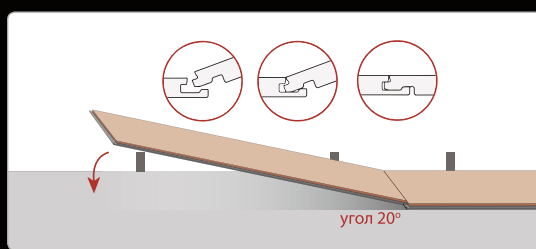
02 МОНТАЖ ВТОРОЙ ПАНЕЛИ
