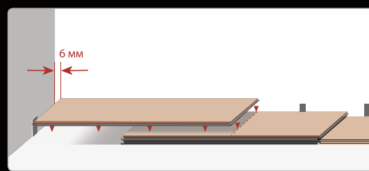
03 МОНТАЖ ПОСЛЕДНЕЙ ДОСКИ 1 РЯДА
